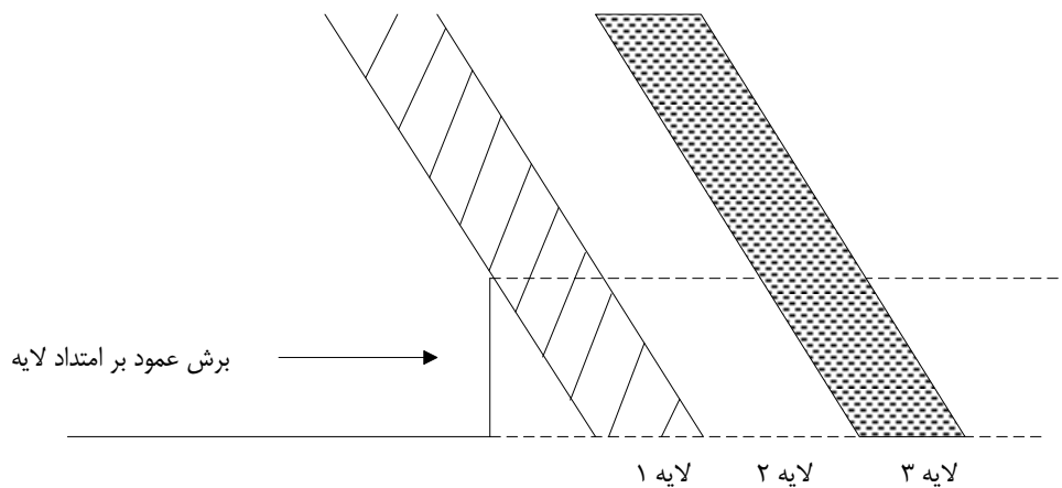
شکل ۲-۴- احداث برش اولیه در لایه‌های مرمريت شیب‌دار
