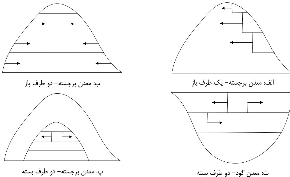
شکل ۴-۴- وضعیت پله‌ها در حالت‌های مختلف
