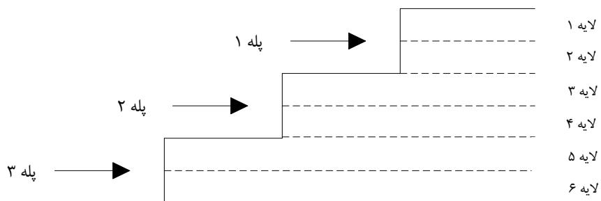
شکل ۲-۳- احداث پله‌های مختلف برای استخراج مرمريت
